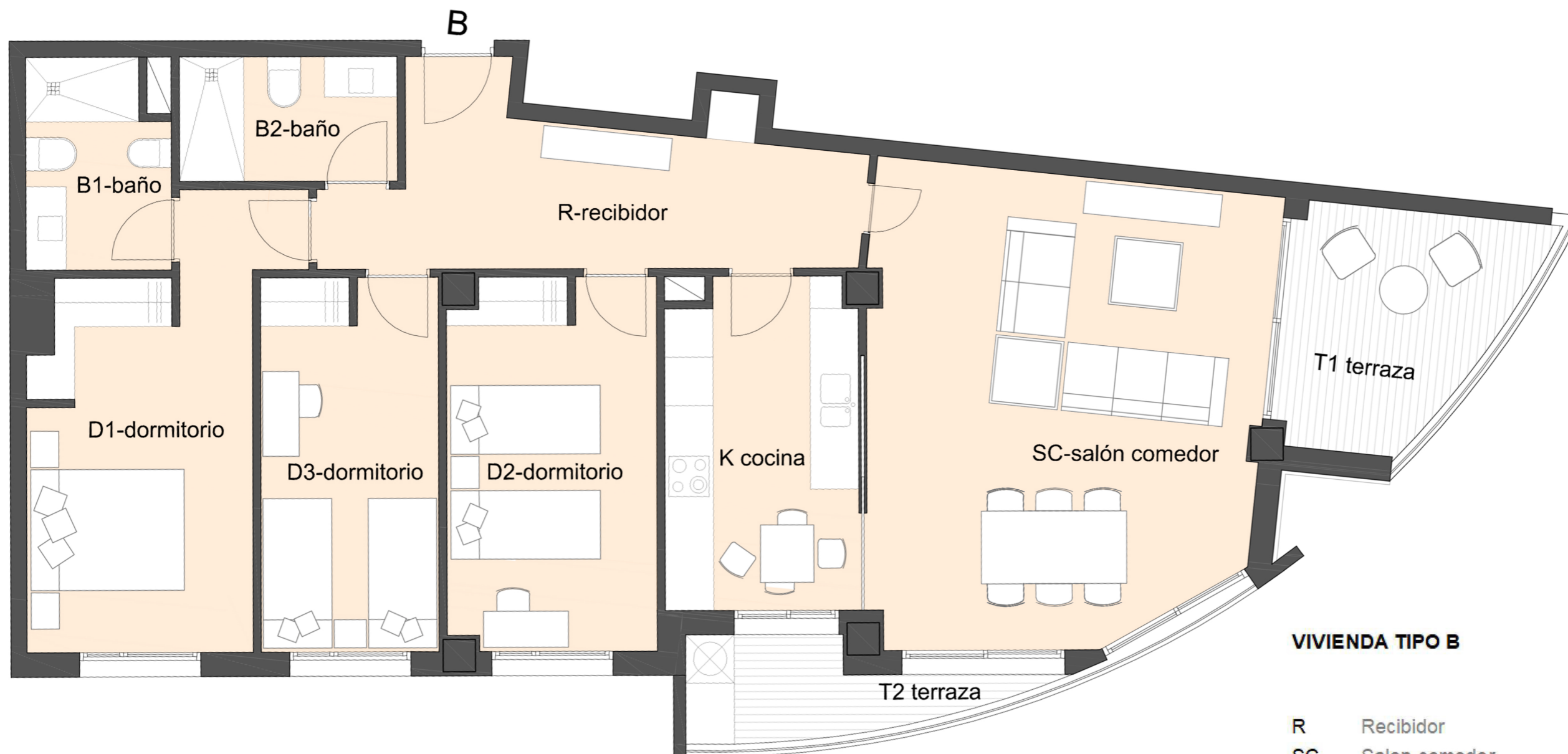
EDIFICIO NEOS VIVIENDA TIPO B ESCALA 1:50
