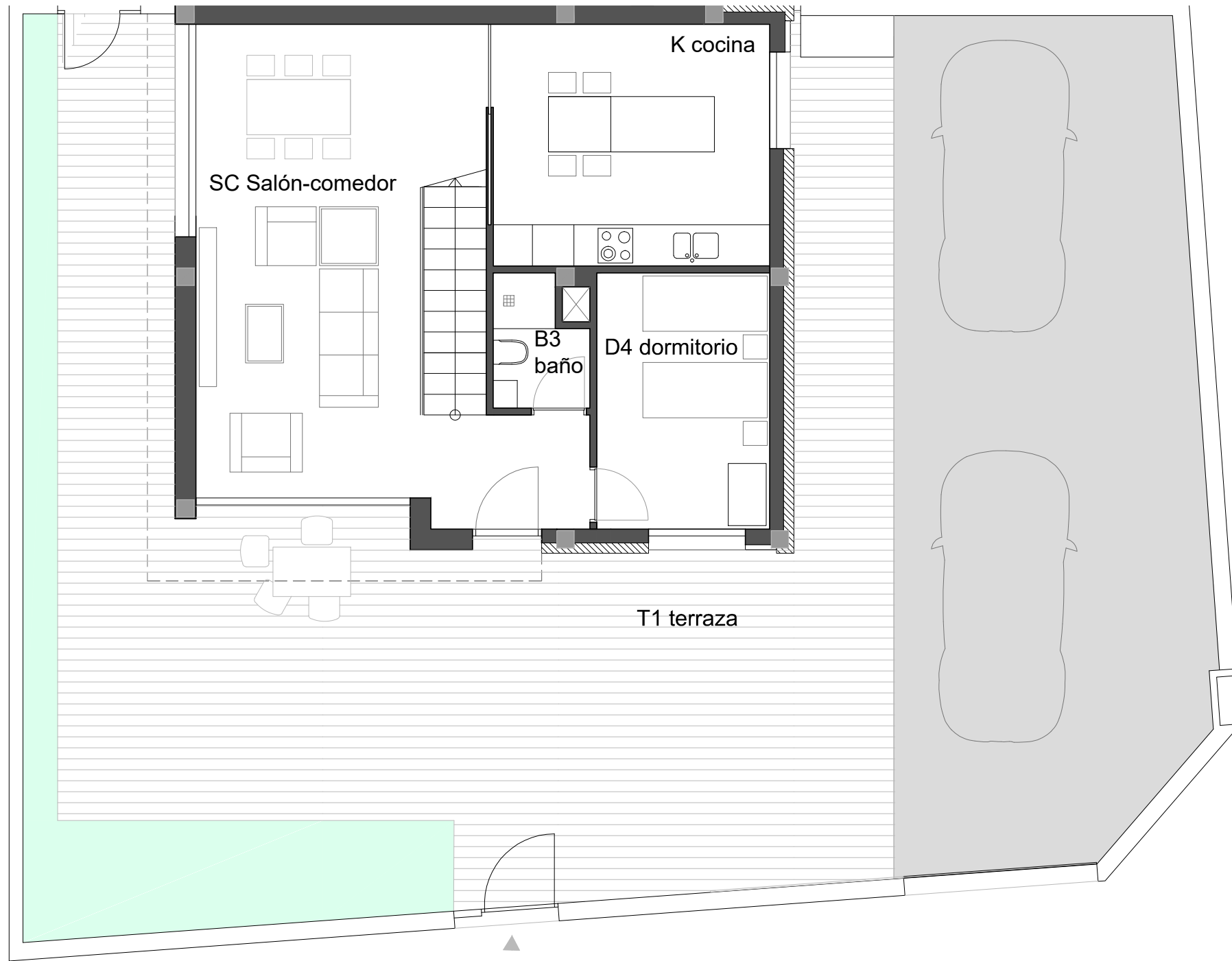
PLANTA BAJA
